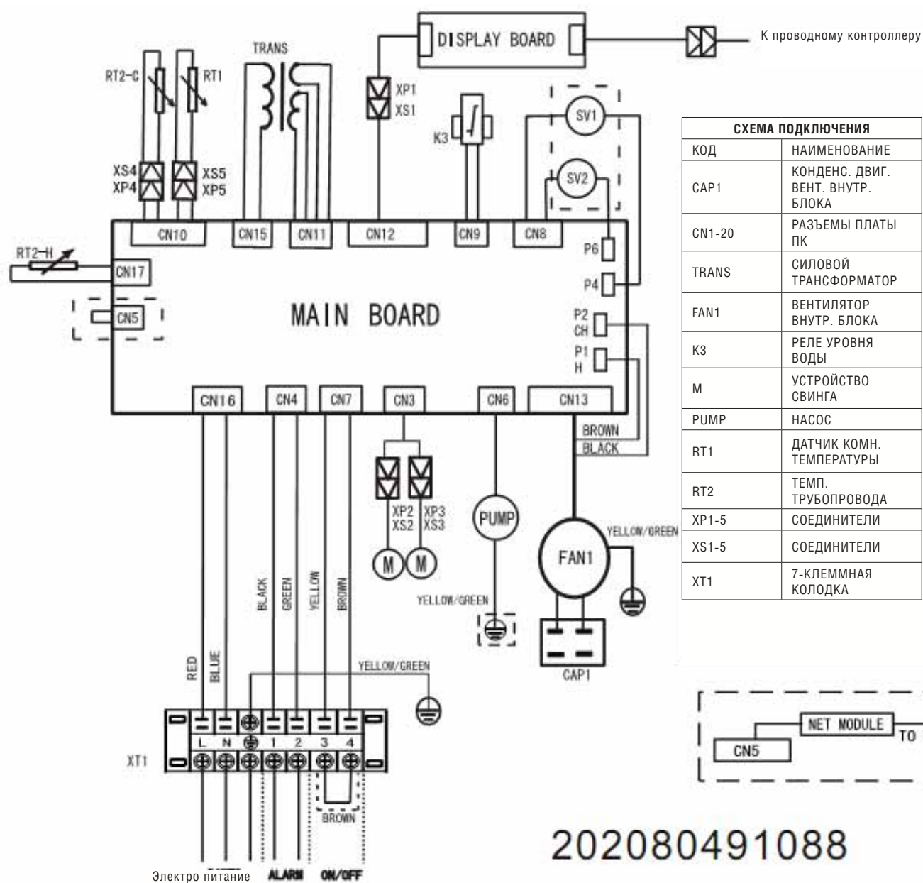
Рис. №4. Электрическая схема агрегатов ACF-60CM4, ACF-70CM4, ACF-105CM4.
