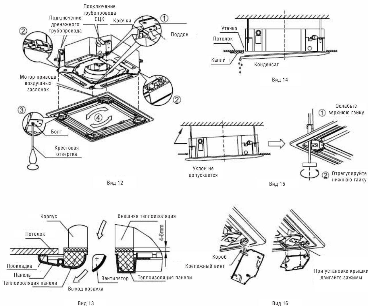
Рис. №9. Установка агрегатов.
