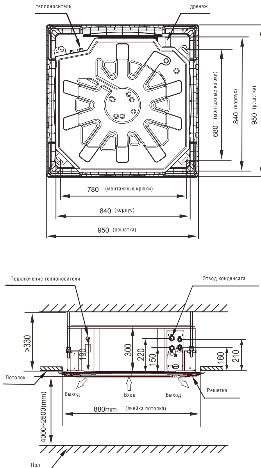
Рис. №1. Габаритные размеры фанкойлов ACF-CM4.
