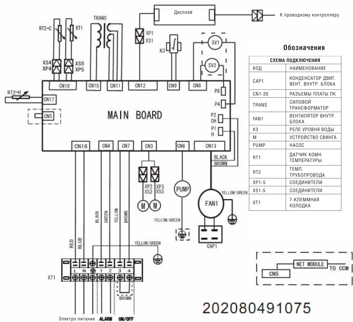
Рис. №3. Электрическая схема агрегатов ACF-50CM4, ACF-65CM4, ACF-95CM4.
