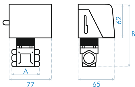
Рис. 1. Размеры
