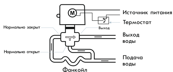
Рис. 4. 3-ходовой клапан
