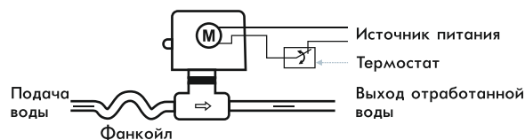
Рис. 3. 2-ходовой клапан
