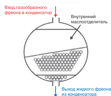
Встроенный маслоотделитель конденсатора
