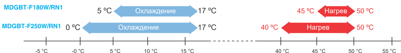
РЕГУЛИРОВКА ТЕМПЕРАТУРЫ ТЕПЛОНОСИТЕЛЯ
