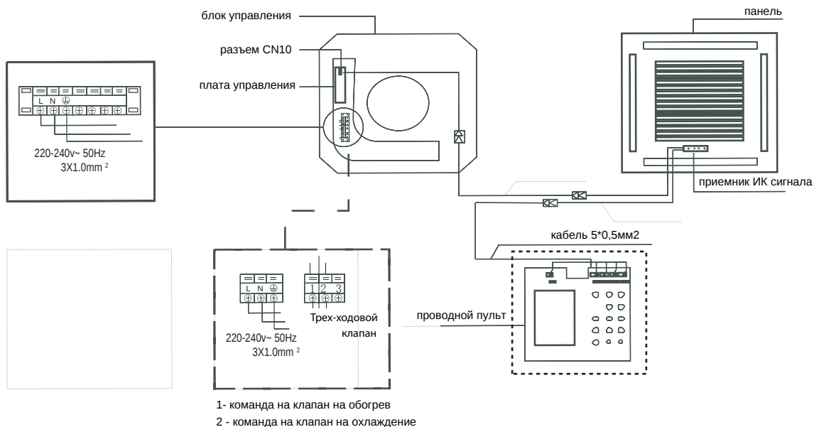
Рисунок №14 Схема электроподключения
