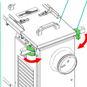
Панель рамы
