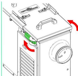
Защелки
